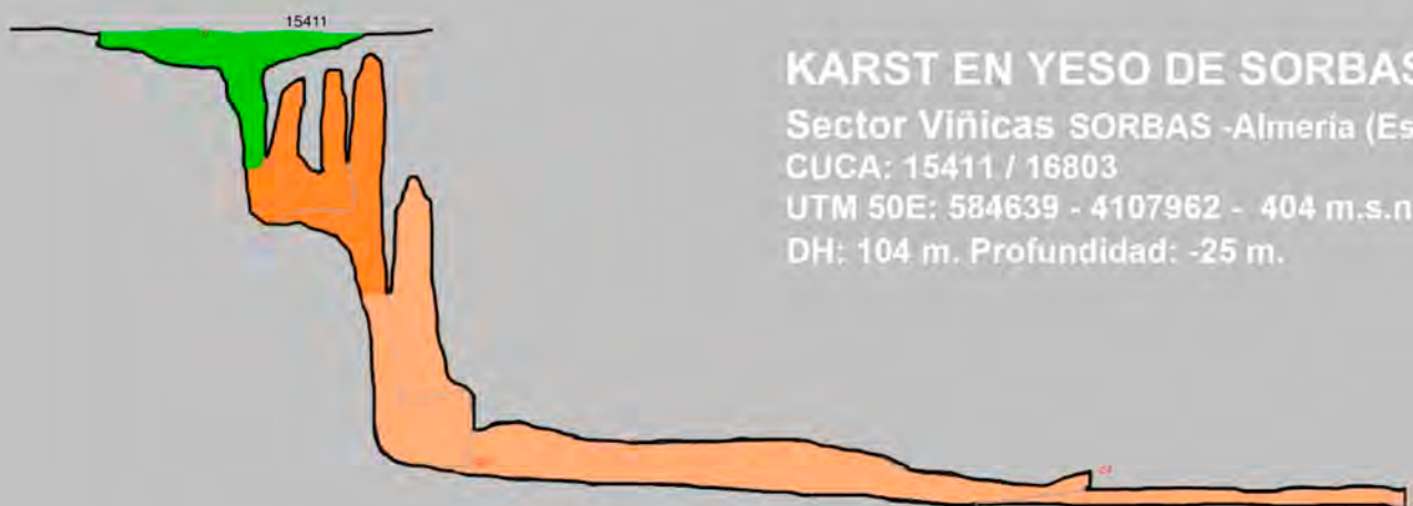
ALZADO
