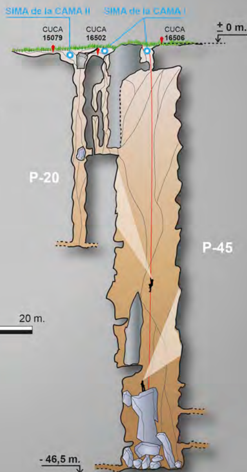
ALZADO DESARROLLADO
