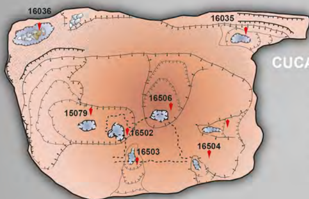
PLANTA DOLINA de la CAMA (Distribución de los CUCAS)
